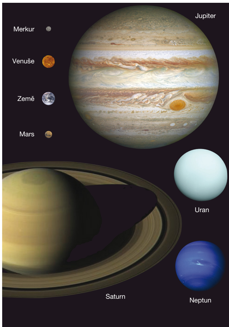
Obrazová příloha 2. Relativní velikosti planet. Jupiter je zhruba 10x větší než Země. Uran a Neptun jsou asi 4x větší než Země. Slunce (není na obrázku) je přibližně 10x větší než Jupiter. Zdroj: NASA/JPL.
